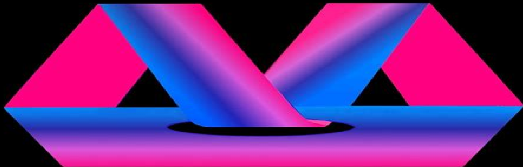
Möbius Strip
