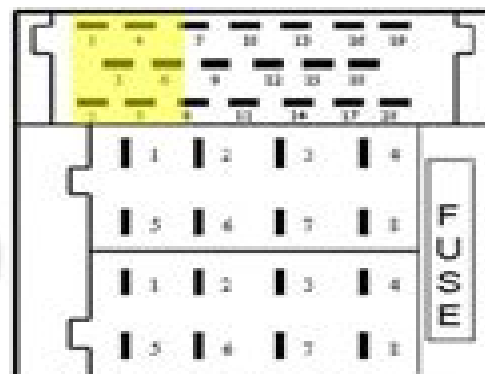
MINI ISO CONNECTOR
