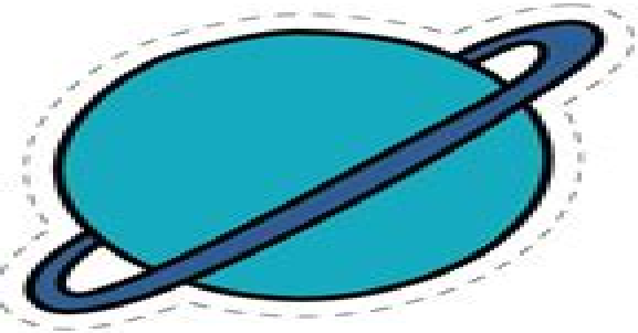
Uranus
